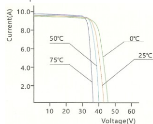
Curva de potência 320W mono I-V a 1000/W/m²
