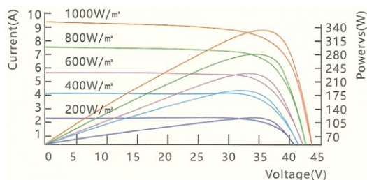
Curva de potência 320W mono I-V a 25°C
