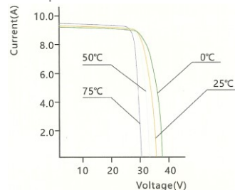
Curva de potência 270W mono I-V a 1000W/m²
