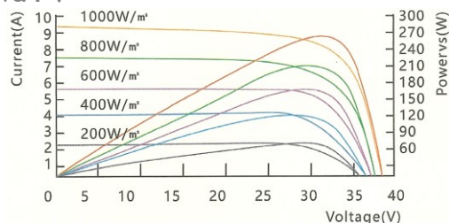
Curva de potência 270W mono I-V a 25°C
