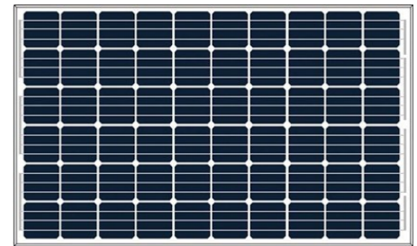
270 - 285 Mono, 1640 x 992mm, 60 células, 4 barramentos, potência desempenho até 17,52%
